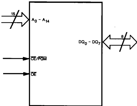
Am27256
