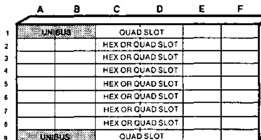
DD11-DK BACKPLANE
