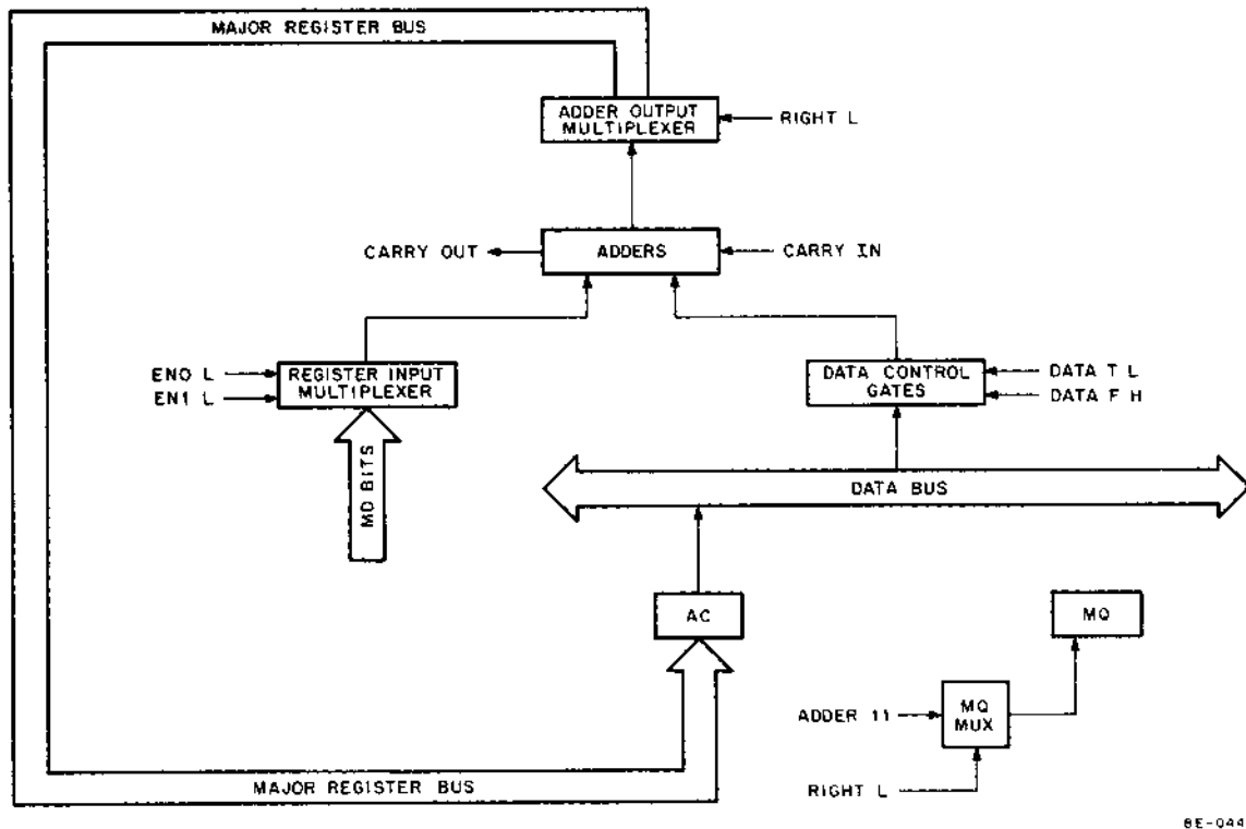
Figure 1-14 MUY Instruction Data Paths
