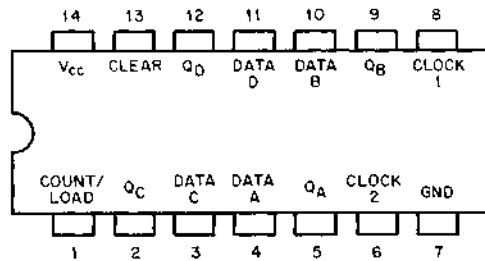
PIN LOCATOR
