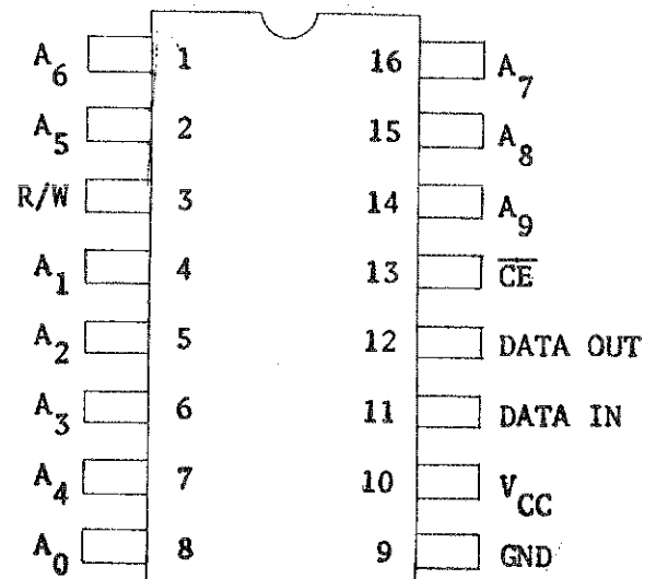
2102A RAM
