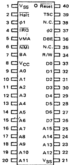
6800 MPU
